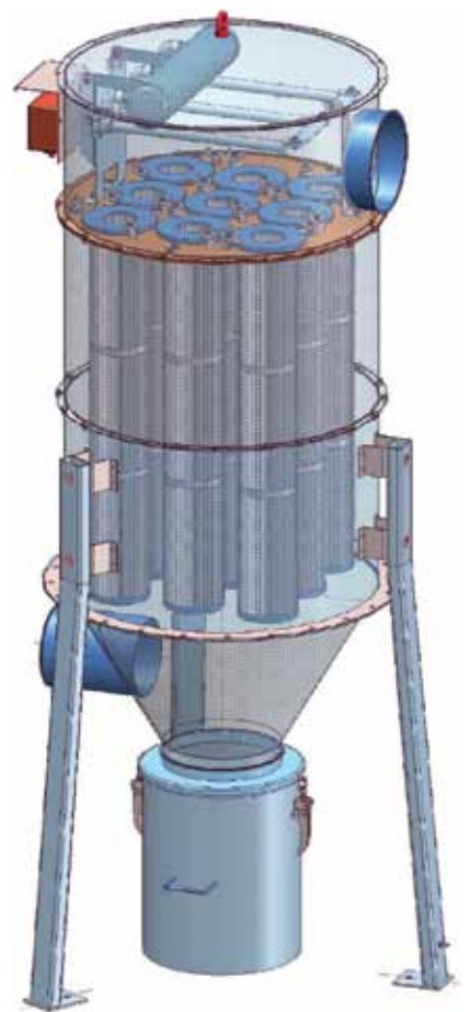
INFA-VARIO-JET, AJV Entstaubungsgerät mit Trichter und Staubsammeltopf
