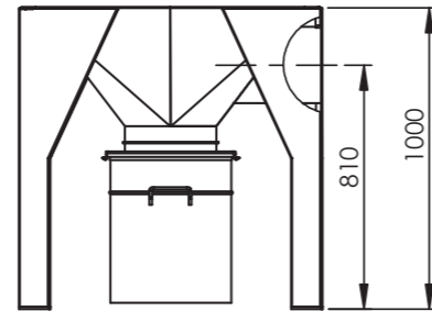
④ Staubaustragstrichter mit Staubsammeltopf Dust hopper with dust bin
