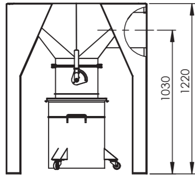
③ Staubaustragstrichter mit Absperrklappe und Staubsammeltopf Dust hopper with butterfly valve and dust bin
