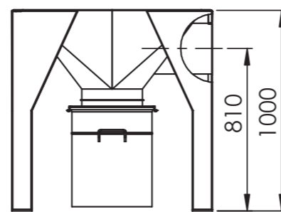
④ Staubaustragstrichter mit Staubsammeltopf Dust hopper with dust bin
