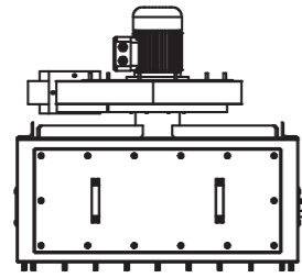
① Ventilator oben Fan on top
