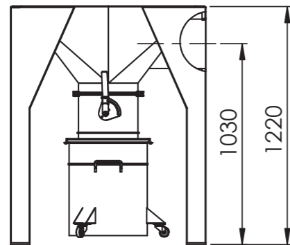
③ Staubaustragstrichter mit Absperrklappe und Staubsammeltopf Dust hopper with butterfly valve and dust bin
